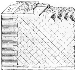
Fig. 508. Structura reticulata.
